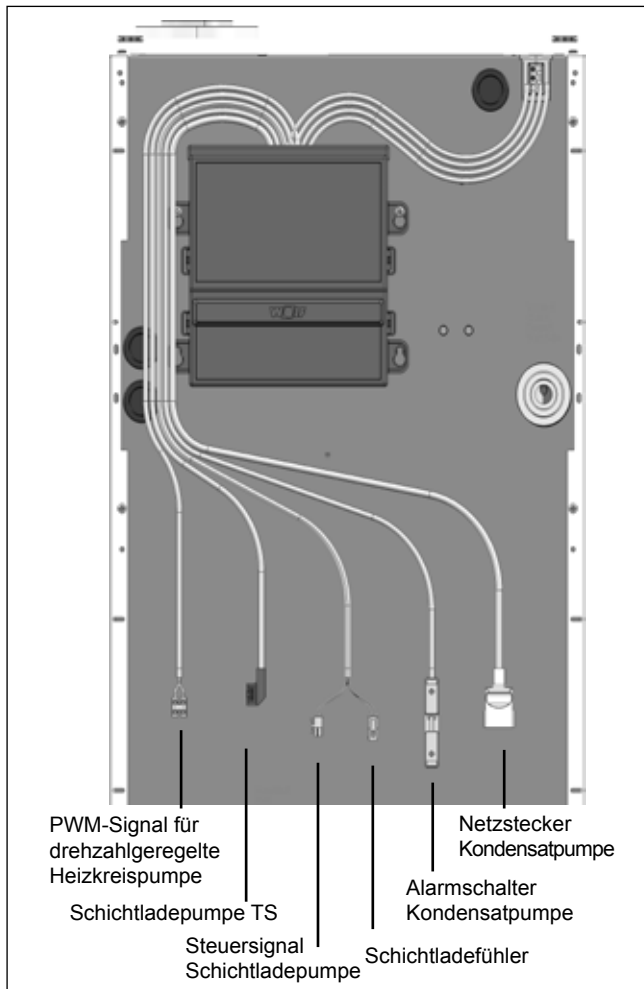
Bild: Elektroanschlusskabel an der Kesselrückseite TOB
