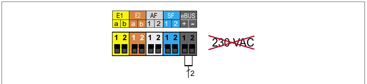
Abb. 5.24 Anschluss WOLF-Regelungszubehör digital (eBus-Schnittstelle)
