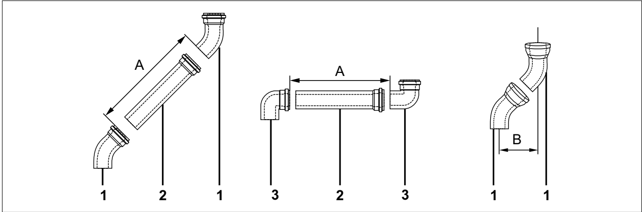
Abb. 5.10 Länge Luft-/Abgasrohr
