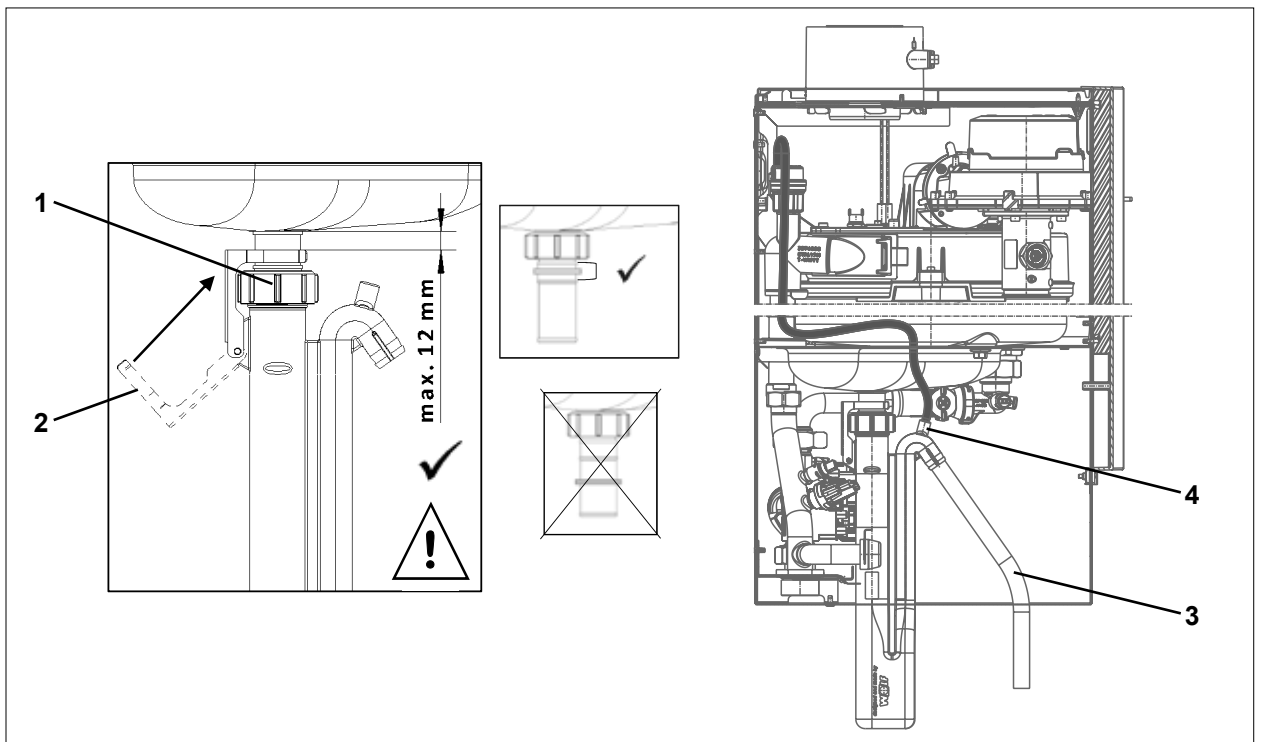
Abb. 5.6 Siphon
