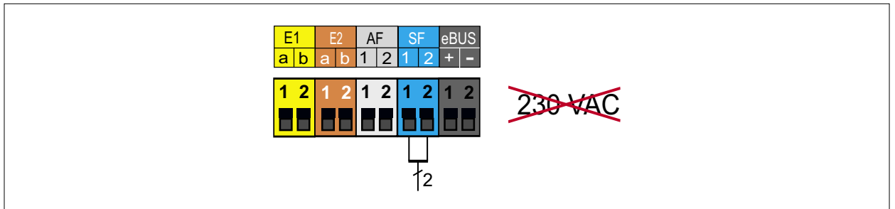
Abb. 5.23 Anschluss Speicherfühler
