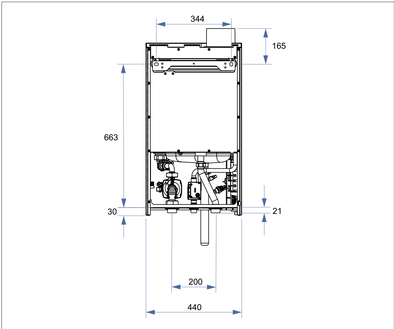
Abb. 11.1 Abmessungen Wärmeezeuger und Anschlüsse in mm
