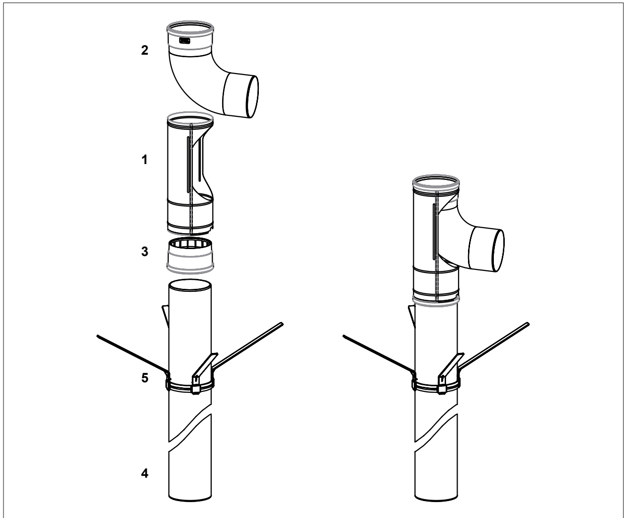
Abb. 4.11 Montage Stützrohr
