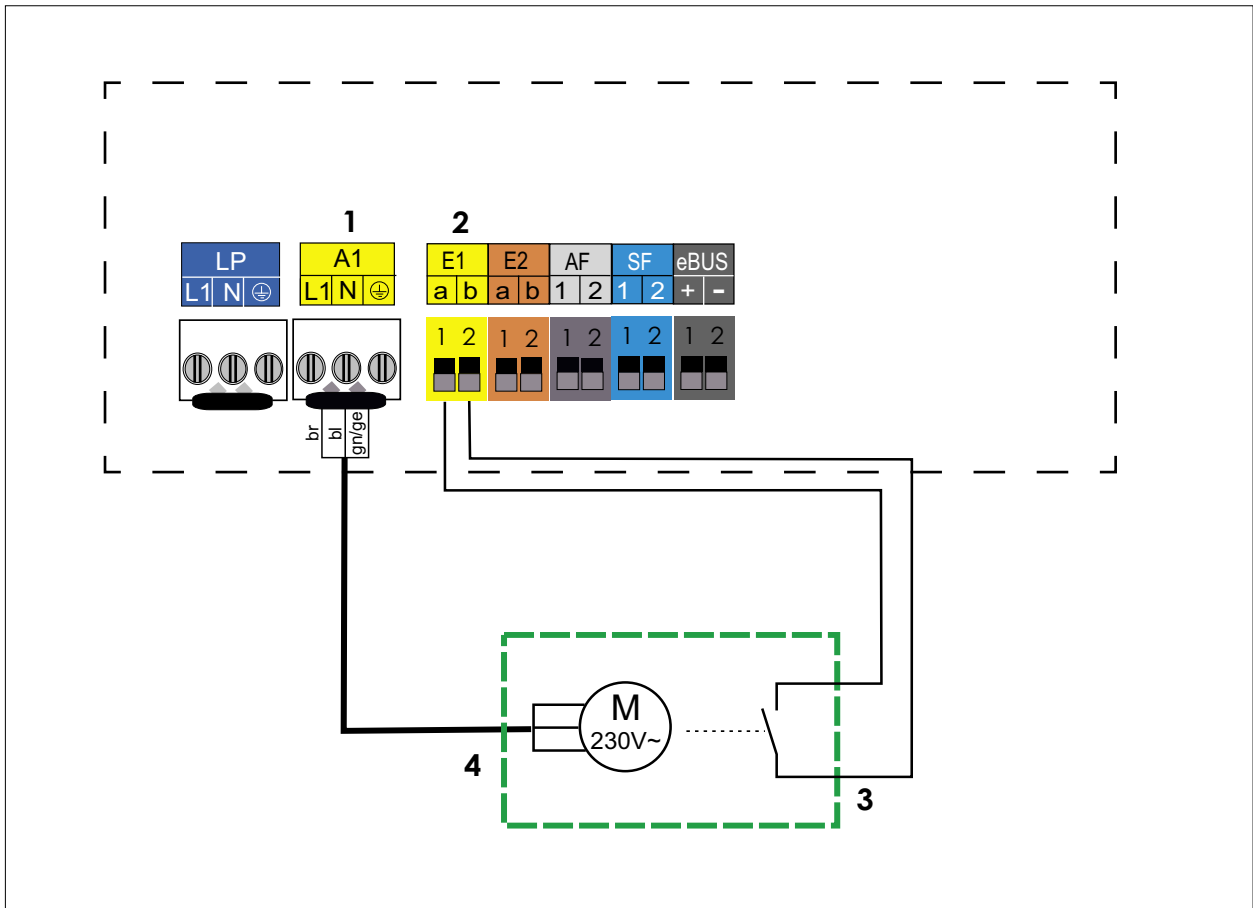
Abb. 5.25 Elektroanschluss Abgasklappe/Zuluftklappe
