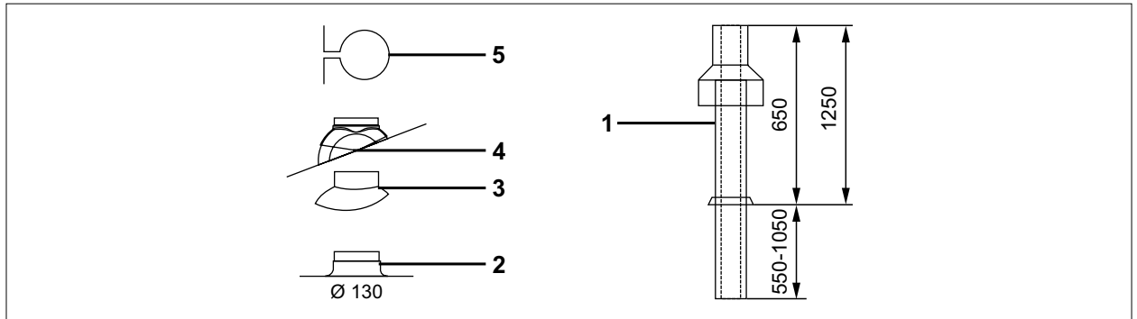
Abb. 5.11 Dachdurchführung [mm]
