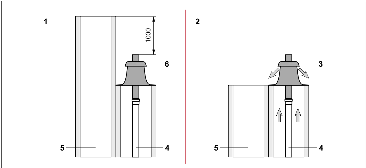
Abb. 4.12 Zweizügiger Schornstein
