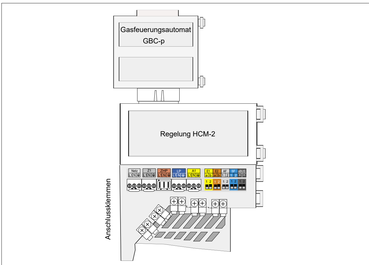
Abb. 5.13 Bauteile Regelung
