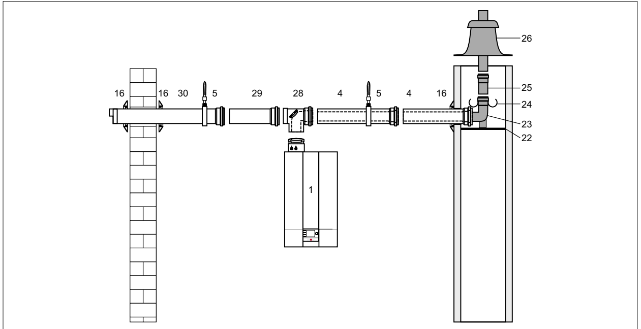
Abb. 4.7 Luft-/Abgasführung waagrecht C83x
