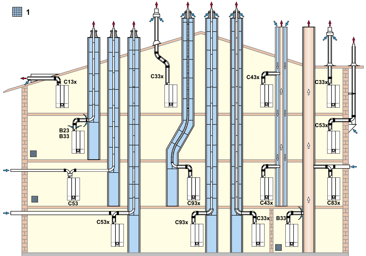
Abb. 4.3 Übersicht Anschlussart
