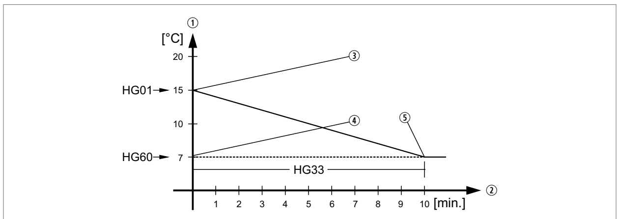
Abb. 7.1 Brennerhysterese
