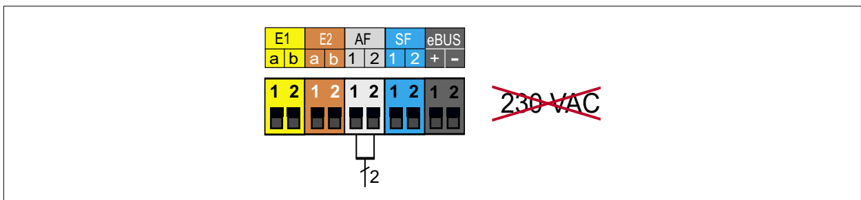
Abb. 5.22 Anschluss Außenfühler
