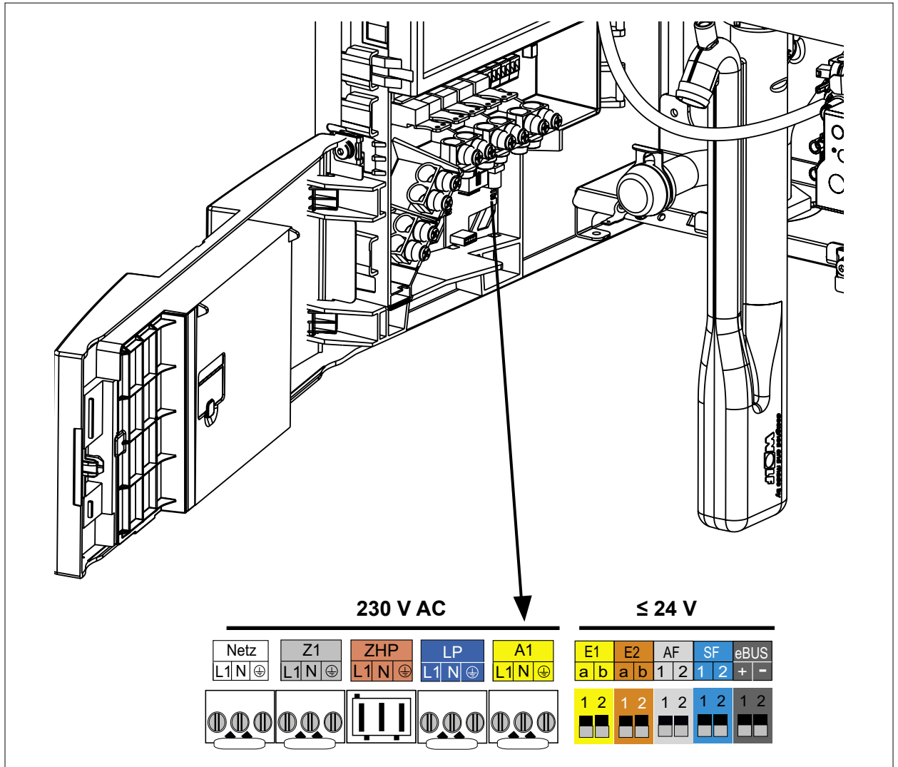
Abb. 5.14 Klemmenbelegung Elektroanschlusskasten
