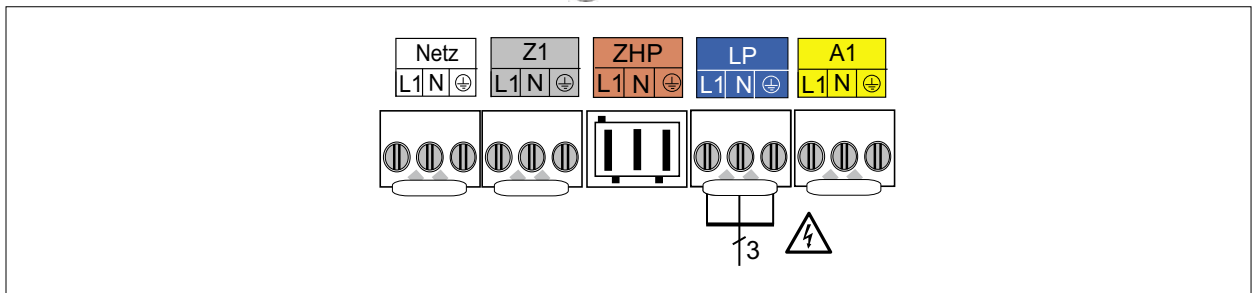
Abb. 5.18 Anschluss Warmwasserladepumpe
