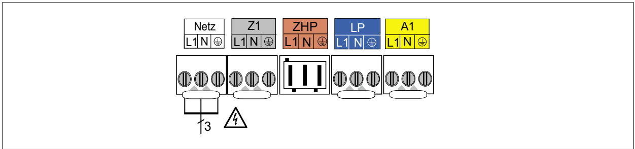
Abb. 5.15 Netzanschluss 230 V
