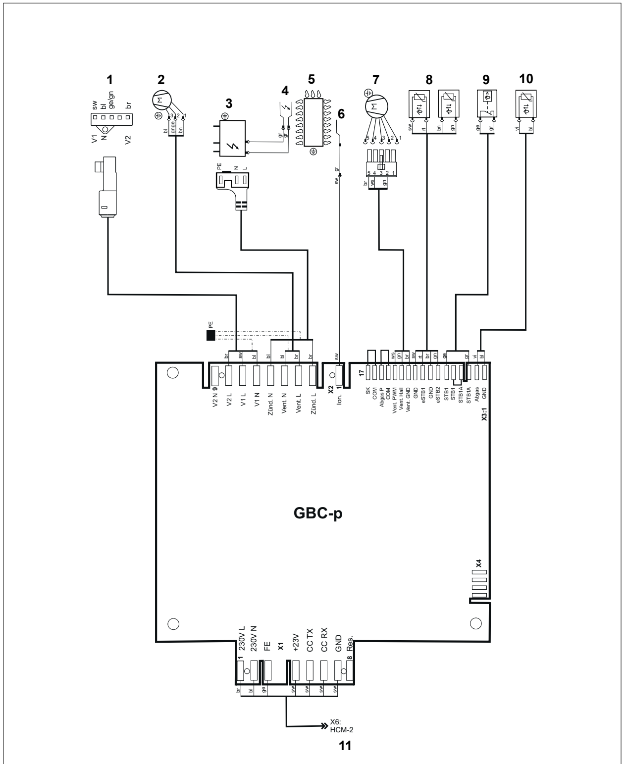
Abb. 12.2 Schaltplan GBC-p
