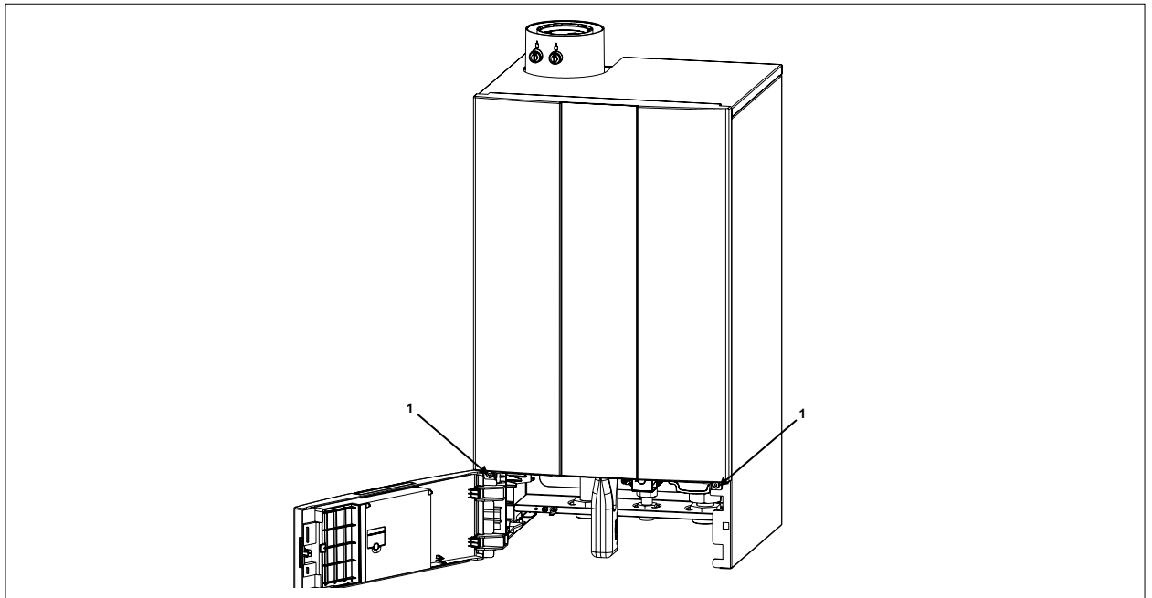
Abb. 5.3 Regelungsdeckel offen
