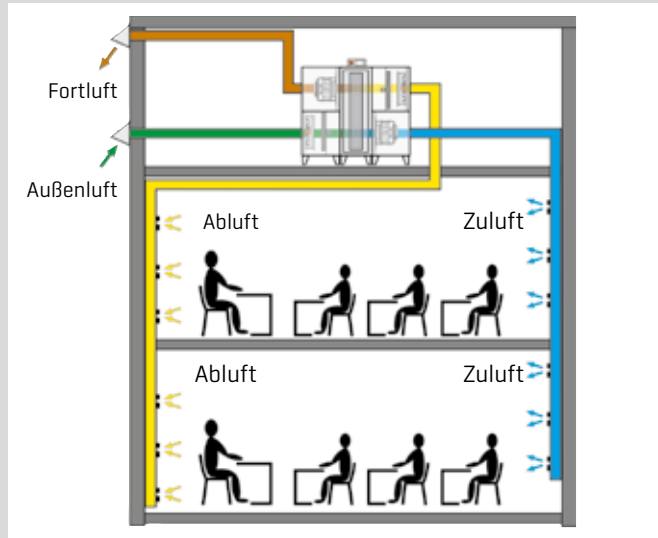
Funktionsdarstellung der Lufteinbringung: CRL-iD
