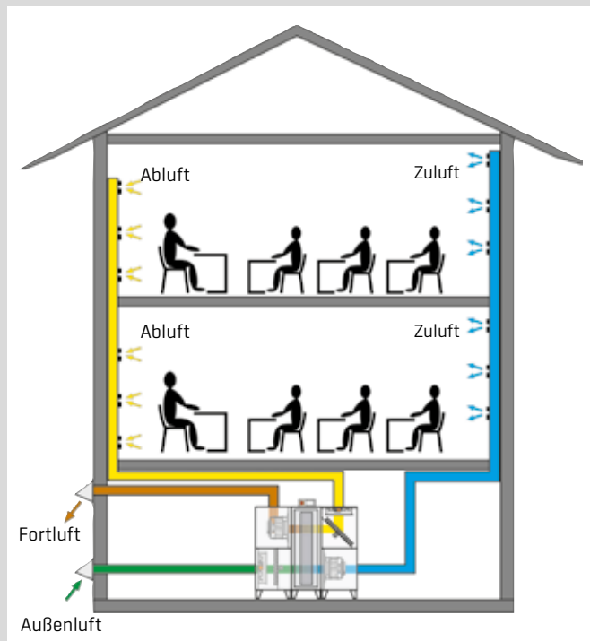
Funktionsdarstellung der Lufteinbringung: CRL-iD
